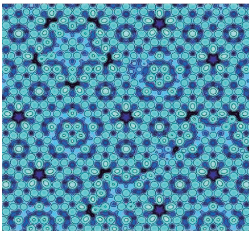
Figura 30. El patrón de un cuasicristal de aleación plata-aluminio (Ag-Al). Las moléculas no se disponen de forma repetitiva, aunque sus pautas forman disposiciones en las que claramente se distingue un orden que se pone de manifiesto en las secuencias de difracción, proporcionadas con simetrías pentagonales, octogonales, icosaédricas y decagonales; estructuras que la tradición consideraba imposibles 29 .
