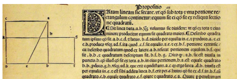
Figura 59. La Proposición II.11 de “Los Elementos” de Euclides contiene el fundamento geométrico de la Sección Áurea.
