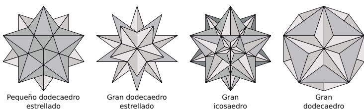
Figura 90. Sólidos de Kepler-Poinsot.
