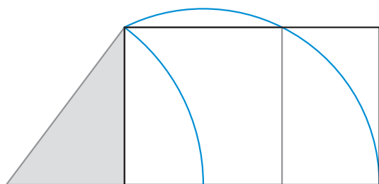
Figura 8. A partir del triángulo 3-4-5.
