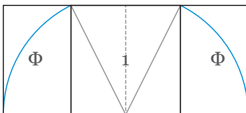
Figura 11. Rectángulo raíz de cinco.
